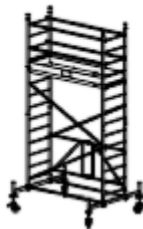
Art nr 920027 Wys.robocza: 4,8m Wys. ruszt.: 3,8m Wys. do pom.: 2,8m
