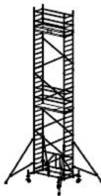
Art nr 920072 Wys. robocza: 9,8m Wys. ruszt.: 8,8m Wys. do pom.: 7,8m
